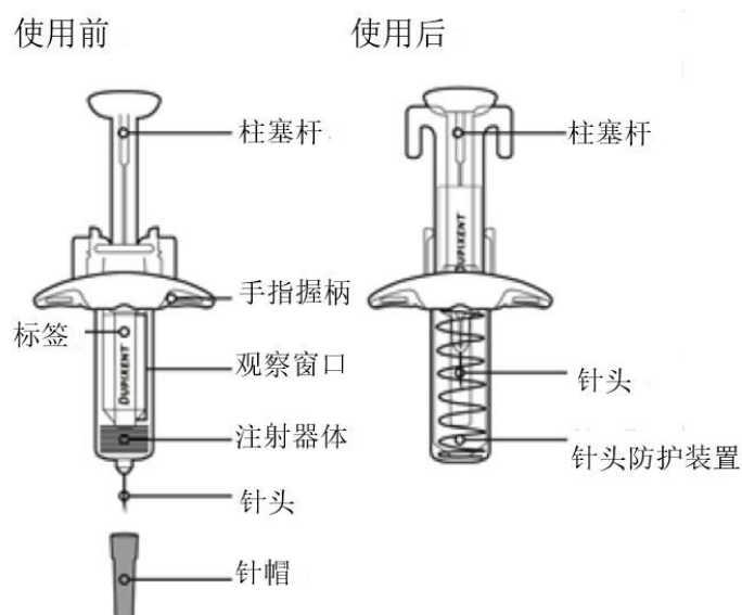
图 1 带有针头防护装置的预充式注射器的示意图
